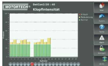
Klopfintensität Visualisierung der Klopfintensität aller überwachten Zylinder. Unterschiedliche Farben informieren über den Systemstatus (normal – Lastreduzierung – kritisch)
