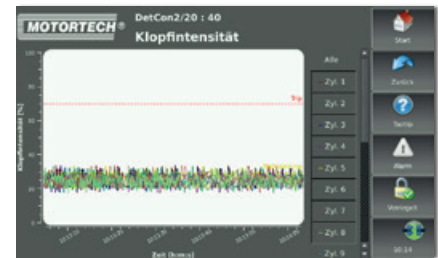
Verlauf der Klopfintensität Visualisierung des Verlaufs der Klopfintensität jedes einzelnen Zylinders
