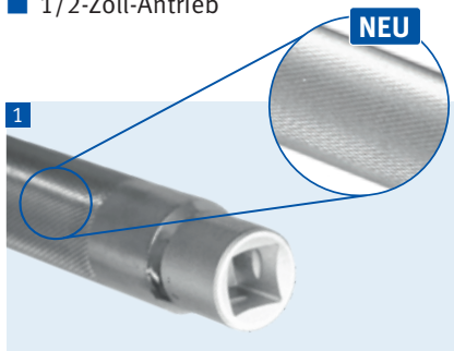
1/2-Zoll-Antrieb und kreuzgerändelte Oberfläche
