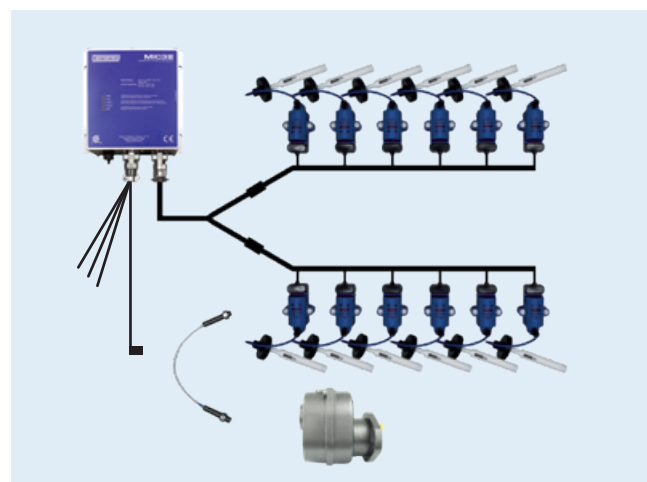
Satz für V-Motoren CATERPILLAR® G3408/G3412
