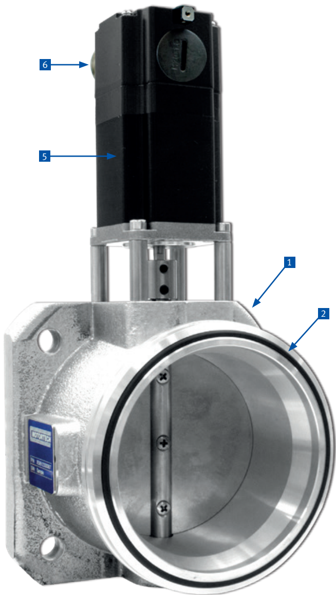
Integrierter Schrittmotor
