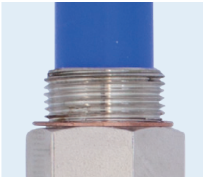
13/16-20-UNEF-Gewinde oben für den Spulenanschluss mit vollen 6 Gewinden gemäß CSA-Anforderungen
